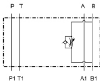
Schaltbild SB
