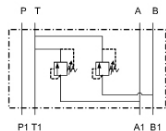
Schaltbild DT
