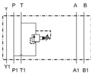
Schaltbild SP
