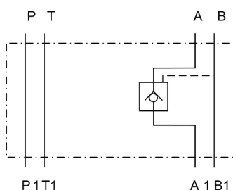
Schaltbild SA
