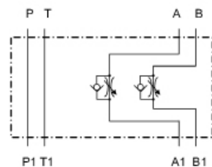
Schaltbild RD
