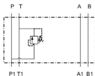
Schaltbild SP
