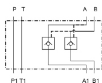
Schaltbild D
