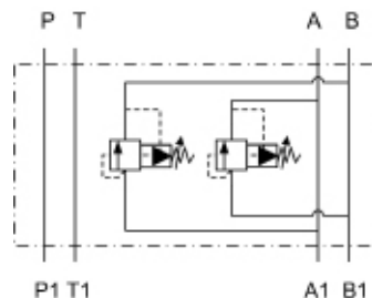
Schaltbild SP
